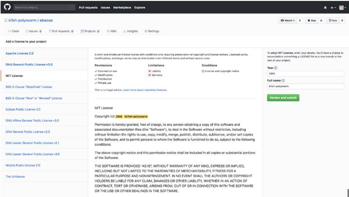
Figure 1.64: MIT License
